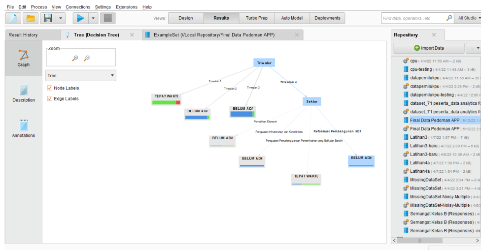
Gambar 2.7 Grafik Pohon
