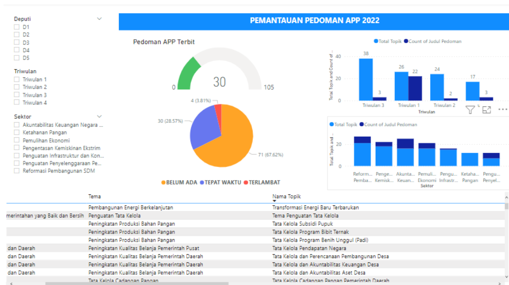
Gambar 2.7 Visualisasi PowerBI
